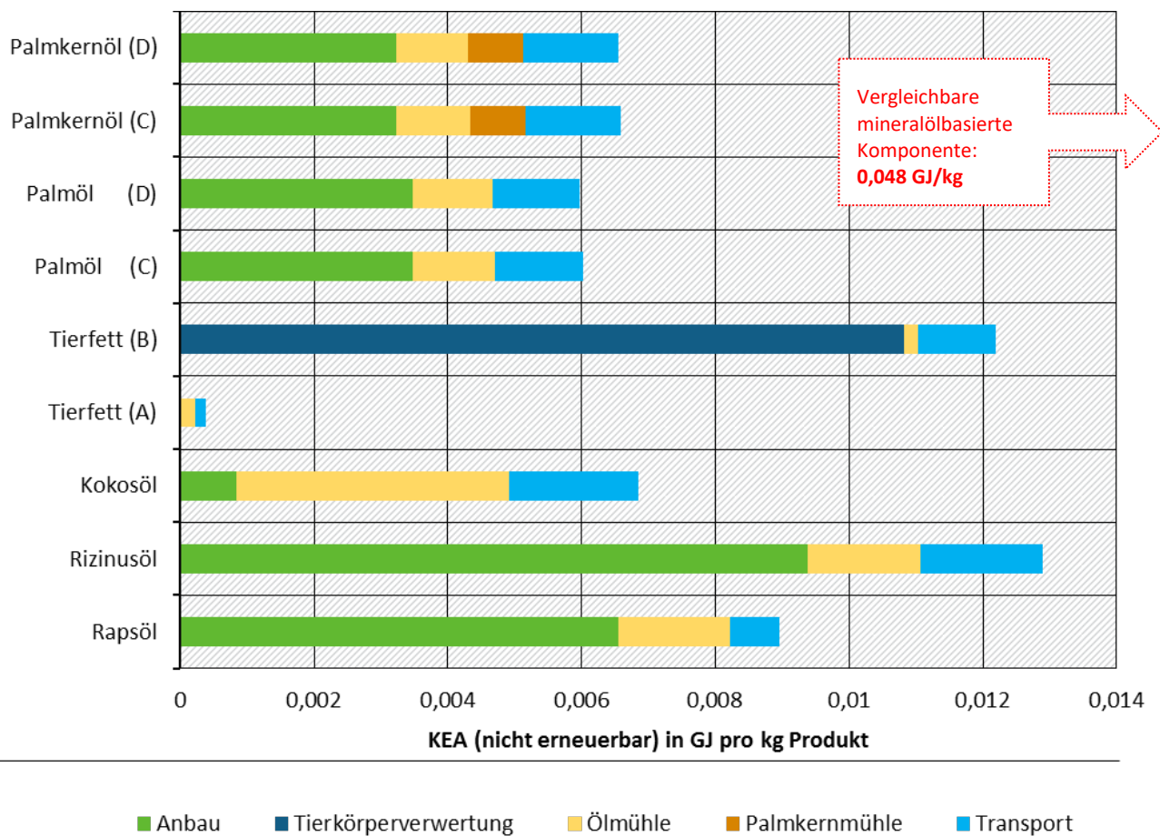
Abbildung 3-3: Kumulierter Energieaufwand (KEA fossil ) für die Herstellung von Pflanzenölen/Tierfetten
