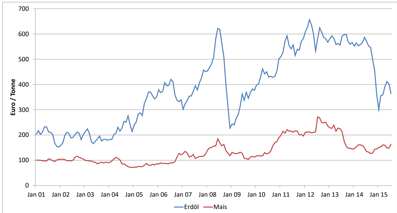
Abbildung 5-2: Preisentwicklung für Erdöl und Körnermais
